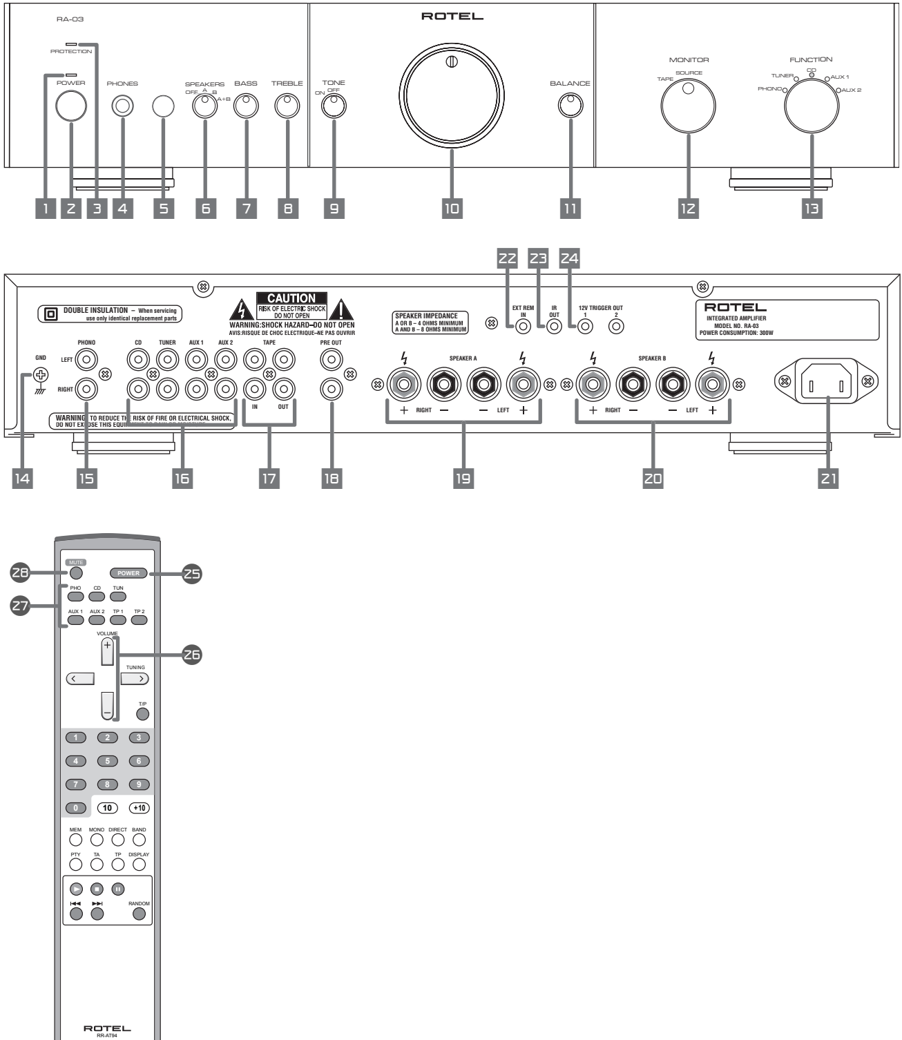
Figure 1: Controls and Connections Commandes et branchements Bedienelemente und Anschlüsse Controlli e collegamenti Controlos y Conexiones De bedieningsorganen en de aansluitingen Funktioner och anslutningar
